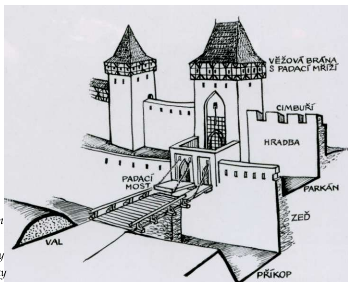
Konstrukční prvky opevnění středověkého hradu
